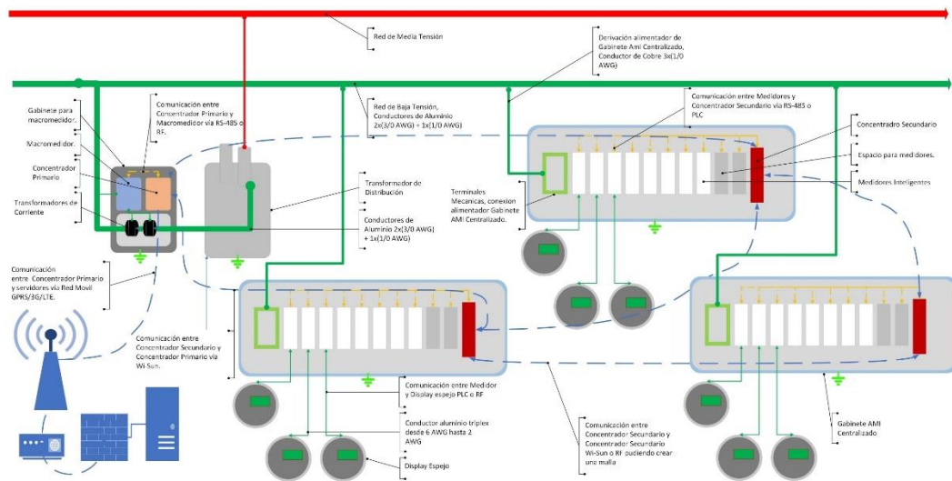
Referencia diagrama de comunicación (Imagen de muestra)
