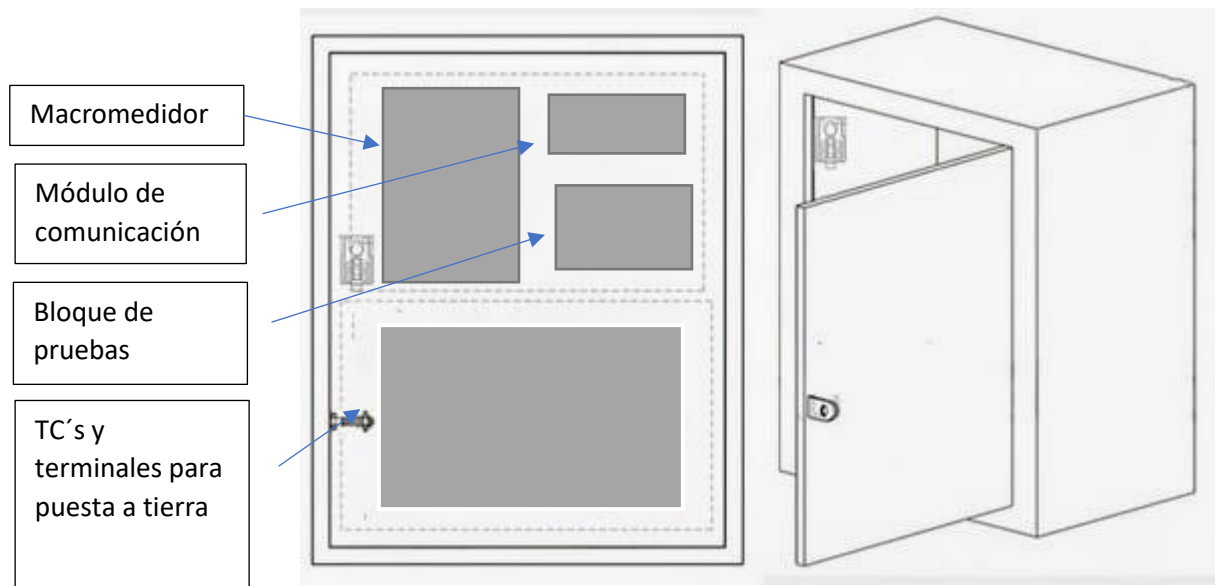
Ilustración 2 Vista Frontal e Isométrica del Gabinete para Macromedidor
